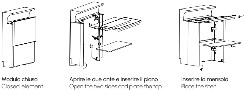
Sistema di montaggio Assembling System
